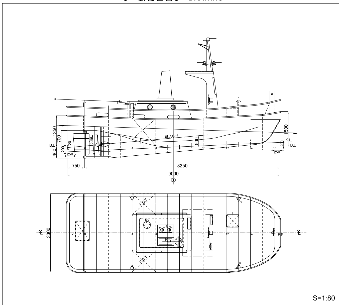
【一般配置図】 DRAWING
